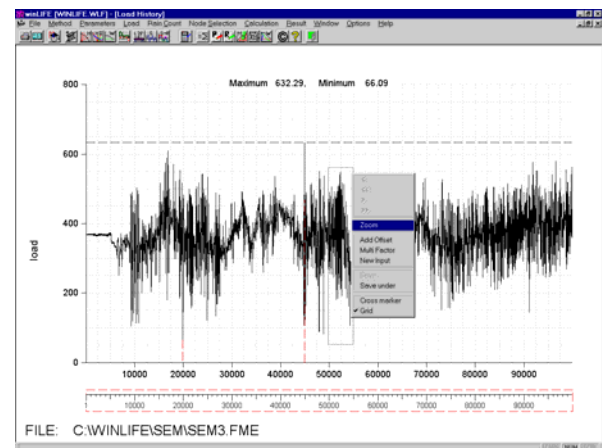
Bild 10: Gemessener Last-Zeit-Verlauf
