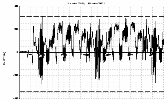
Bild 12: gemessene Last des Bauteils über der Zeit
